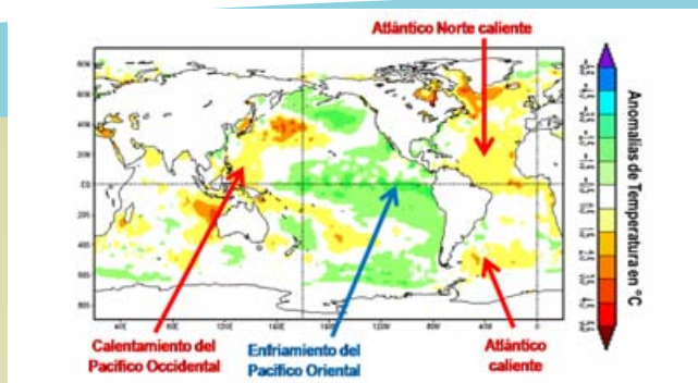
Anomalías globales de temperatura del mar a mediados de Noviembre de 2010. (Fuente CMB/NOAA)
